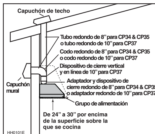
INSTALACIÓN HABITUAL DE LOS TUBOS, MODELOS CP34 Y CP35 (UN SOLO VENTILADOR) O CP37 (DOBLE VENTILADOR)
