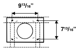
VUE DE HAUT DU CADRE CROISÉ
