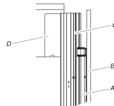
A. Porte du réfrigérateur B. Panneau de porte pleine grandeur C. Garniture latérale D. Support de grille
