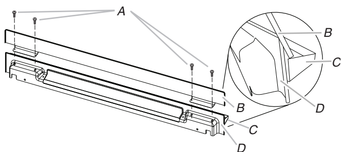
A. Vis n° 8-18 x 1/4" C. Pièce d'évent supérieure B. Garniture de l'évent inférieur D. Pièce d'évent inférieur
