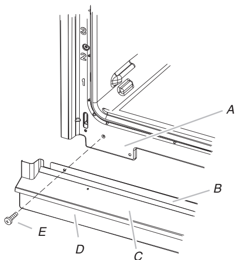
A. Châssis du four D. Garniture de l'évent inférieur B. Support de l'évent E. Vis n° 8-18 x 3/8" C. Évent du four
