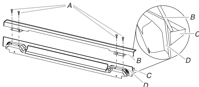
A. Vis n° 8-18 x 1/4" C. Pièce d'évent supérieure B. Déflecteur du tiroir-réchaud D. Pièce d'évent inférieur
