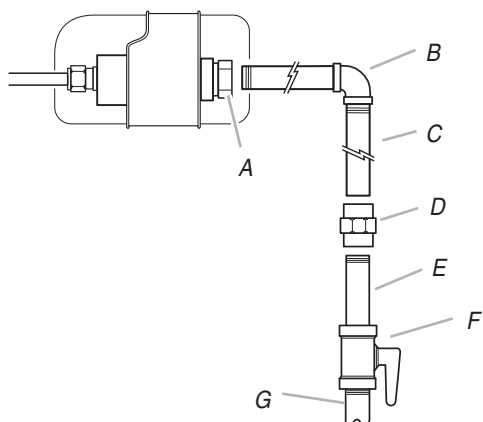
A. Raccord à compression du détendeur B. Coude à 90° C. Tuyau en fer noir D. Raccord droit E. Raccord droit F. Robinet d'arrêt manuel G. Tuyau de gaz de 1/2" ou 3/4"
