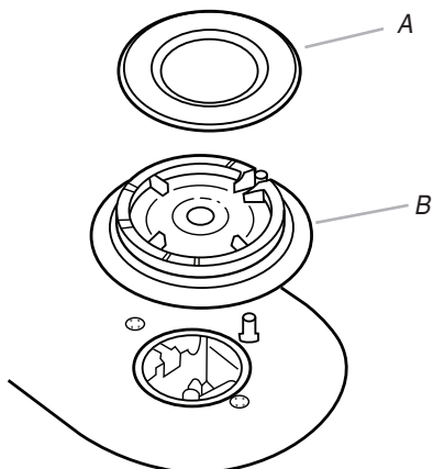
A. Chapeau de brûleur B. Brûleur
