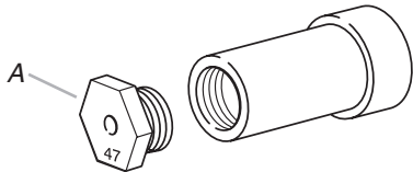
A. Gicleur pour gaz naturel portant la mention "47".
