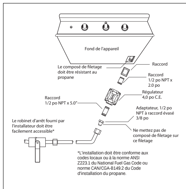
FIG. 22 Gaz naturel
