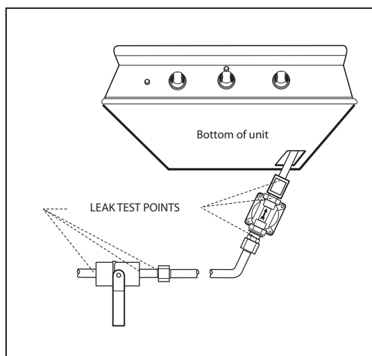
FIG. 31 Nat. Gas
