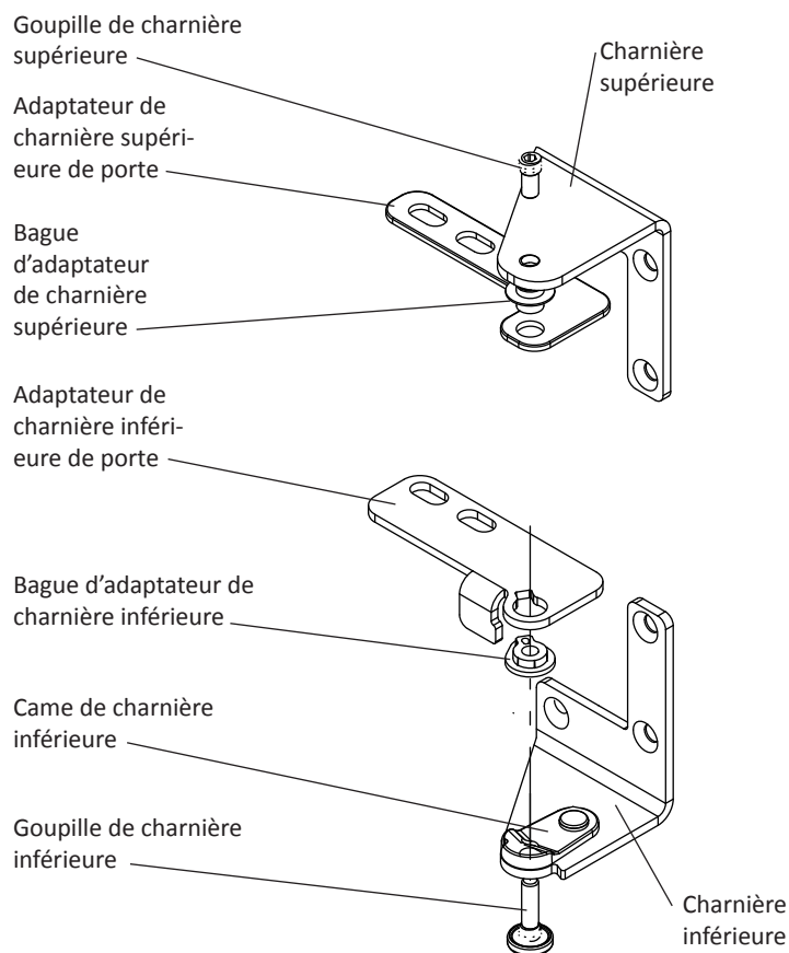
Figure 12 Charnières montrées du côté droit
