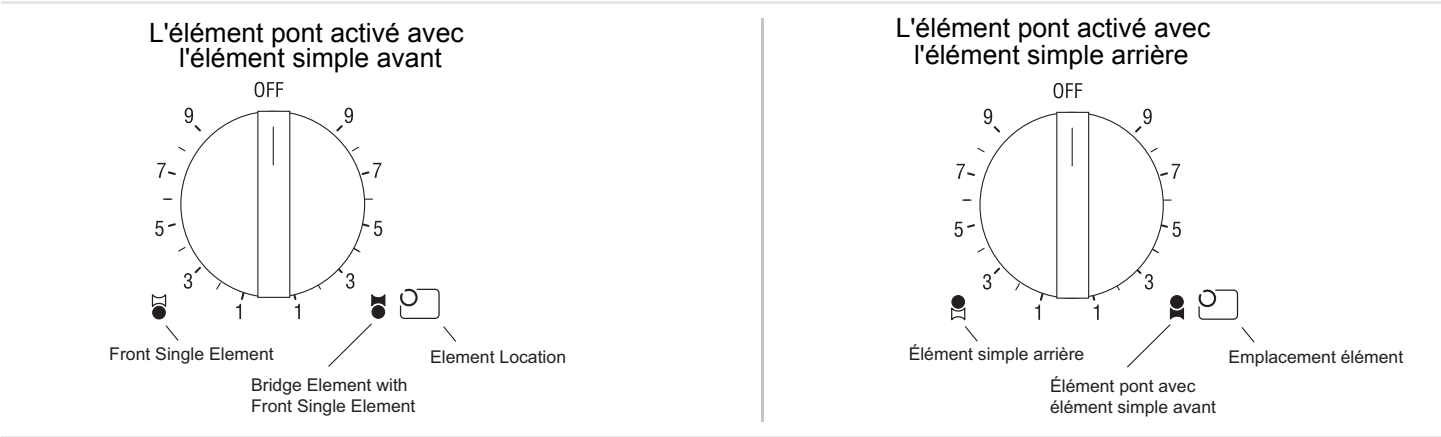
Figure 12: Bouton d'élément pon
