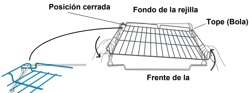
Figura 6: Reensamblado
