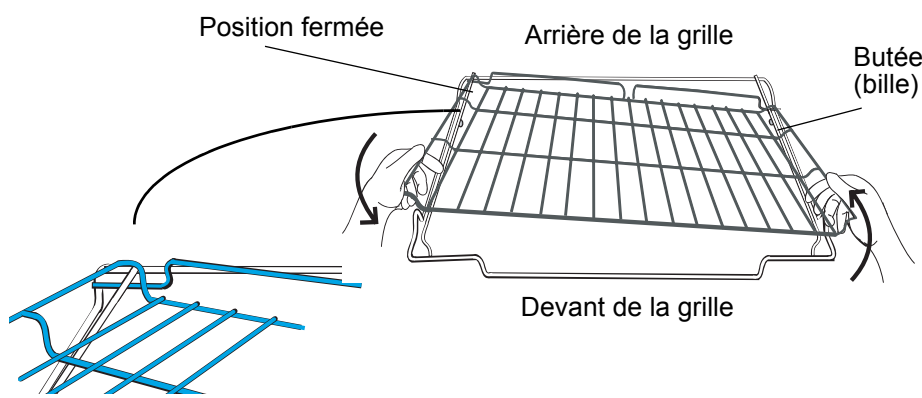
Figure 6: Réassemblage
