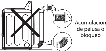
Conductor demasiado largo o muy torcido Tubería demasiado larga o con demasiados codos
