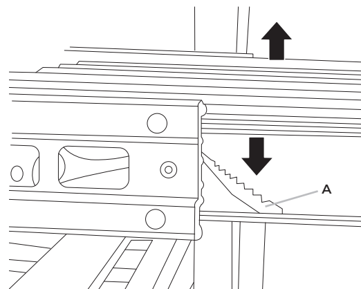
A. Levier
