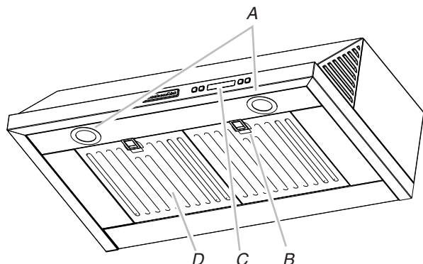
A. Logements des lampes à halogène B. Poignée du plateau à graisse C. Commandes du ventilateur et de l'éclairage D. Filtre à graisse
