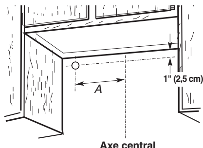
A. 12" (30,5 cm) pour les modèles de 30" (76,2 cm) 12¼" (31,1 cm) pour les modèles de 36" (91,4 cm)
