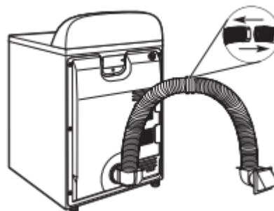
Installation par le dessus (Aussi possible avec un coude décalé)
