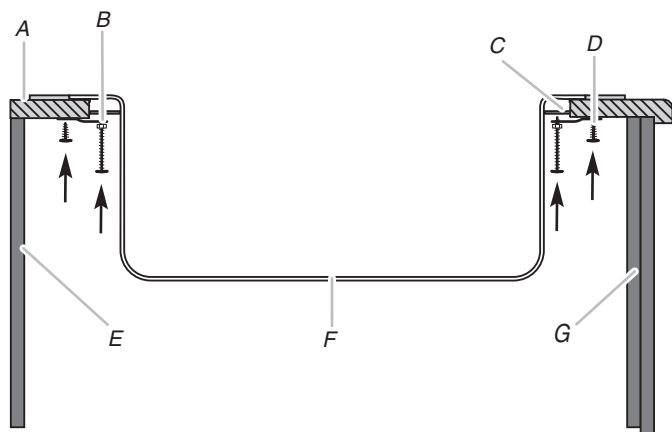
A. Plan de travail B. Vis C. Bride de serrage D. Vis du plan de travail (non fournies) E. Montants du meuble F. Évier G. Face avant du meuble
