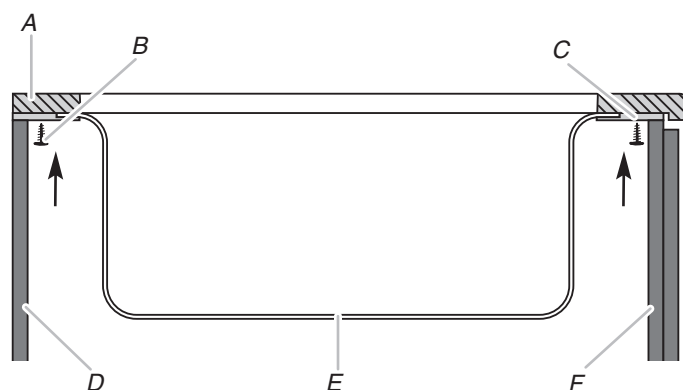
A. Plan de travail B. Vis C. Bride de serrage D. Montants du meuble E. Évier F. Face avant du meuble
