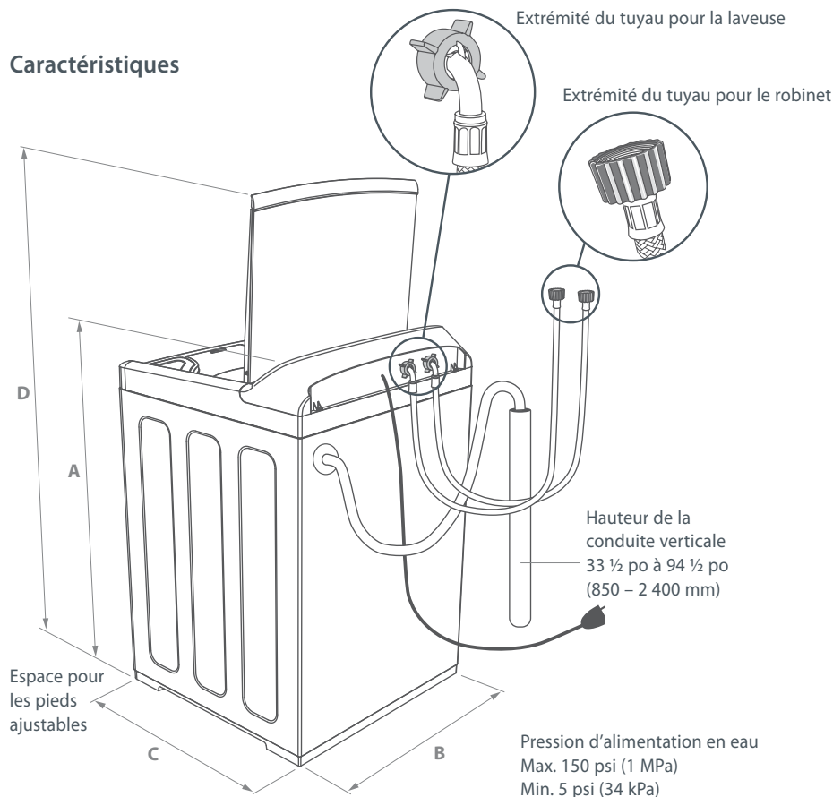
Fig.2 Dimensions et raccords de la laveuse
