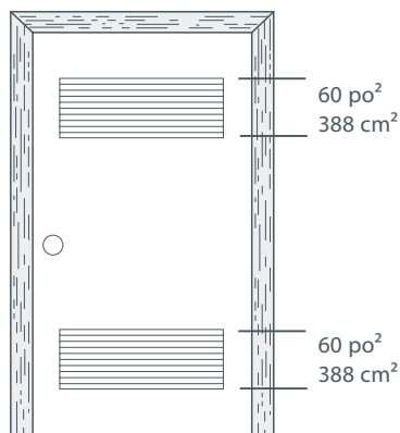
Fig.11 Porte-persienne pour laveuse et sécheuse
