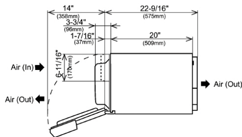
Top Dimensions
