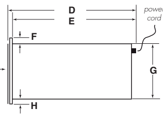
WDUI-30 DIMENSIONS Side View
